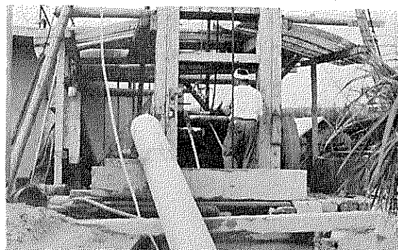
深さ135メートルの大住水源のさく井工事(写真は工事中のもの)
